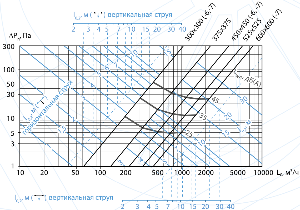
Аэродинамические и акустические характеристики диффузоров 4АПН-С, 4АПР-С при подаче воздуха в помещение комбинированными струями: горизонтальной настилающей и вертикальной прямоточной
