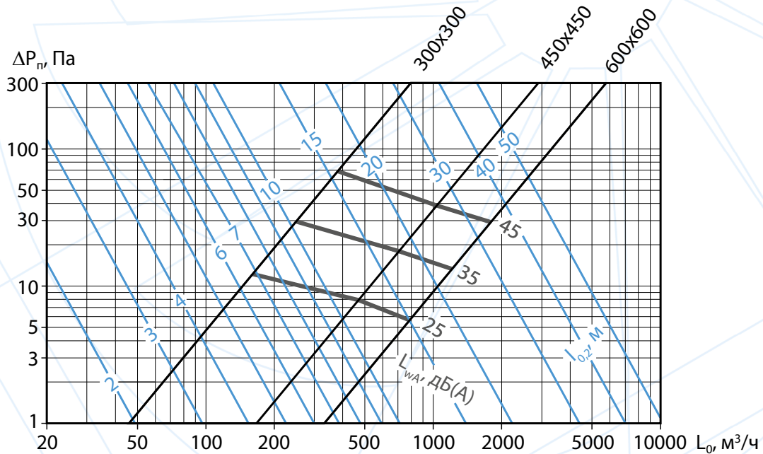
Аэродинамические и акустические характеристики диффузоров 2АПНу, 2АПРу при подаче воздуха в помещение двусторонними настилающимися струями
