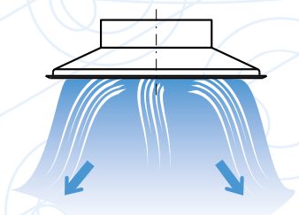
Схемы струй, формируемых диффузорами ДКУ(Т), ДКК(Т), 1ДКФ, 2ДКФ
