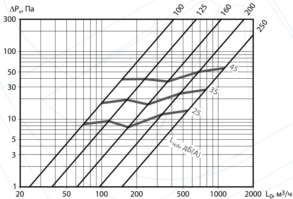
Аэродинамические и акустические характеристики ДПУ-М при удалении воздуха из помещения
