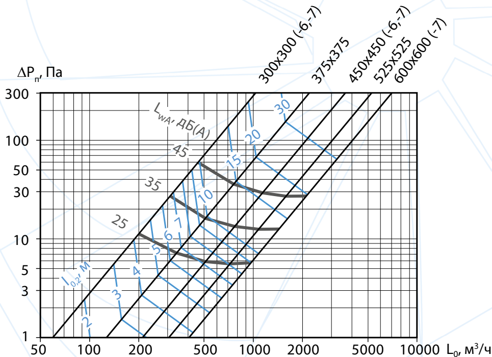
Аэродинамические и акустические характеристики диффузоров 4АПН-П, 4АПР-П при подаче воздуха в помещение комбинированными струями (горизонтальной настилающейся и вертикальной прямоточной)
