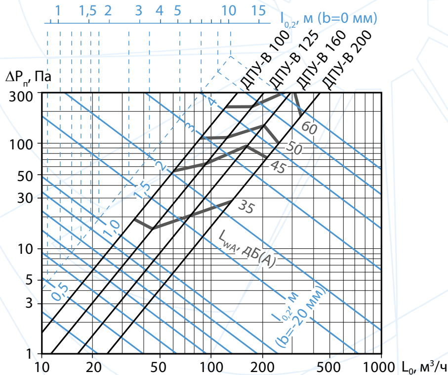
Аэродинамические и акустические характеристики ДПУ-В при подаче воздуха в помещение
