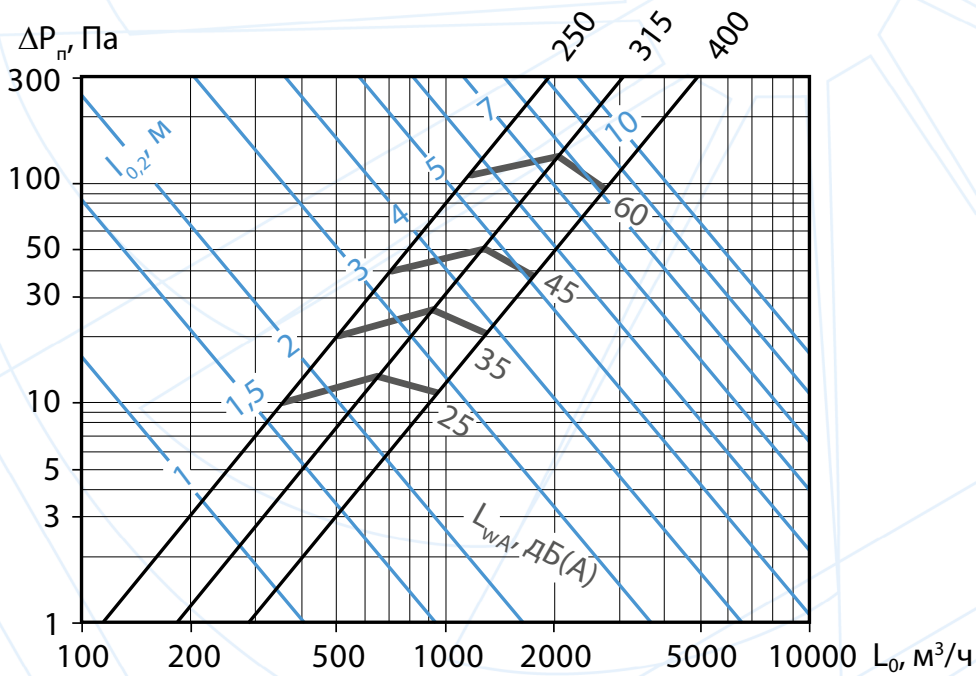
Аэродинамические и акустические характеристики ДКП (коническая струя) при подаче воздуха в помещение при наличии и отсутствии настилаящей поверхности
