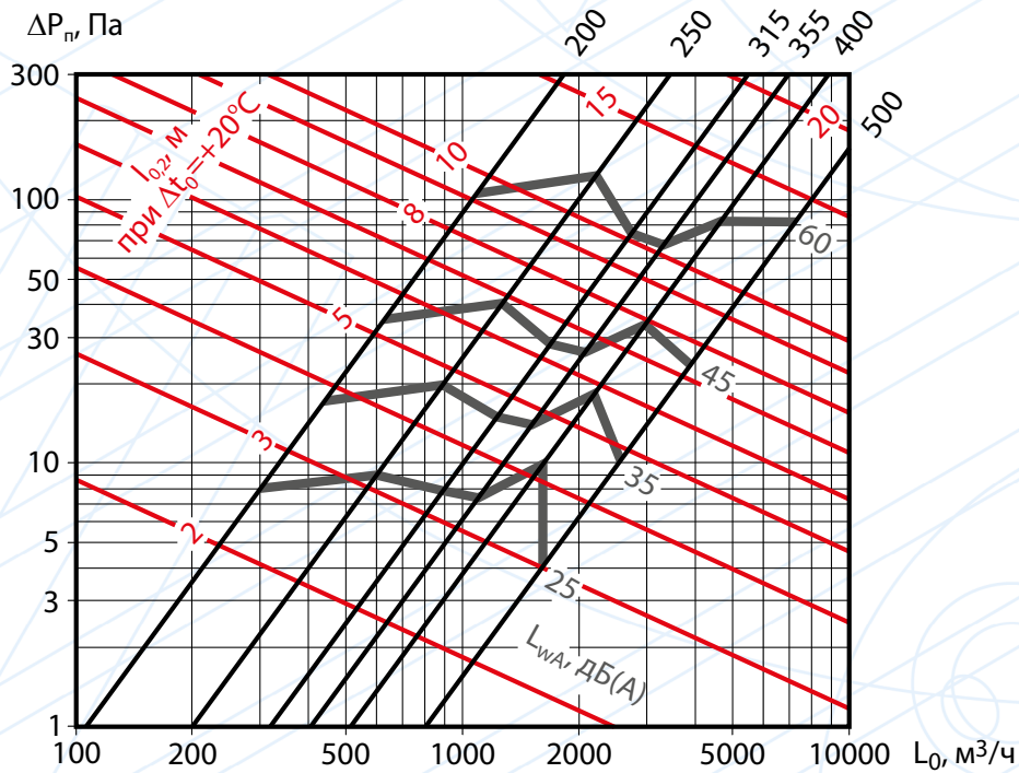
Аэродинамические и акустические характеристики ДКВ-Т при подаче воздуха в помещение неизотермической ( \Delta t_0 = +20^\circ\text{C} ) вертикальной компактной струей при \alpha=0^\circ
