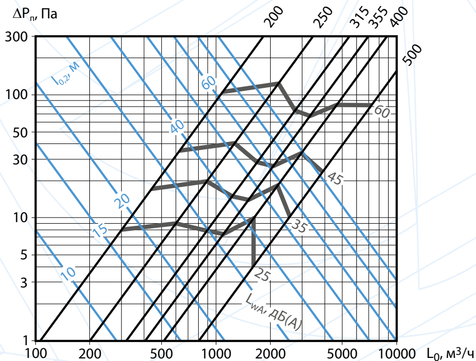
Аэродинамические и акустические характеристики ДКВ при подаче воздуха в помещение компактной струей при угле наклона лопаток \alpha=0^\circ
