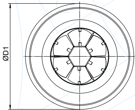
а) ДКВ с ручной регулировкой
