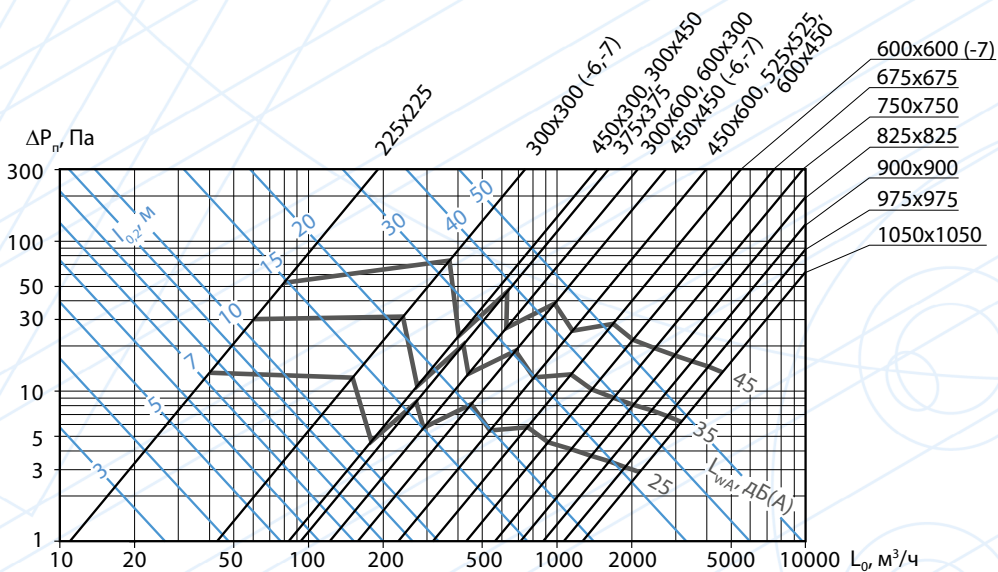
Аэродинамические и акустические характеристики диффузоров 1АПН, 1АПР при подаче воздуха в помещение односторонними настилающимися струями
