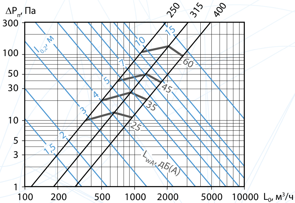
Аэродинамические и акустические характеристики ДКП (веерная настилаящая часть струи) при подаче воздуха в помещение комбинированными струями при наличии настилаящей поверхности
