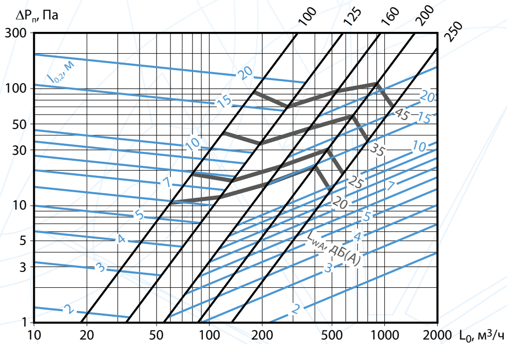
Аэродинамические и акустические характеристики ДПУ-М при подаче воздуха в помещение вертикальной конической смыкающейся струей
