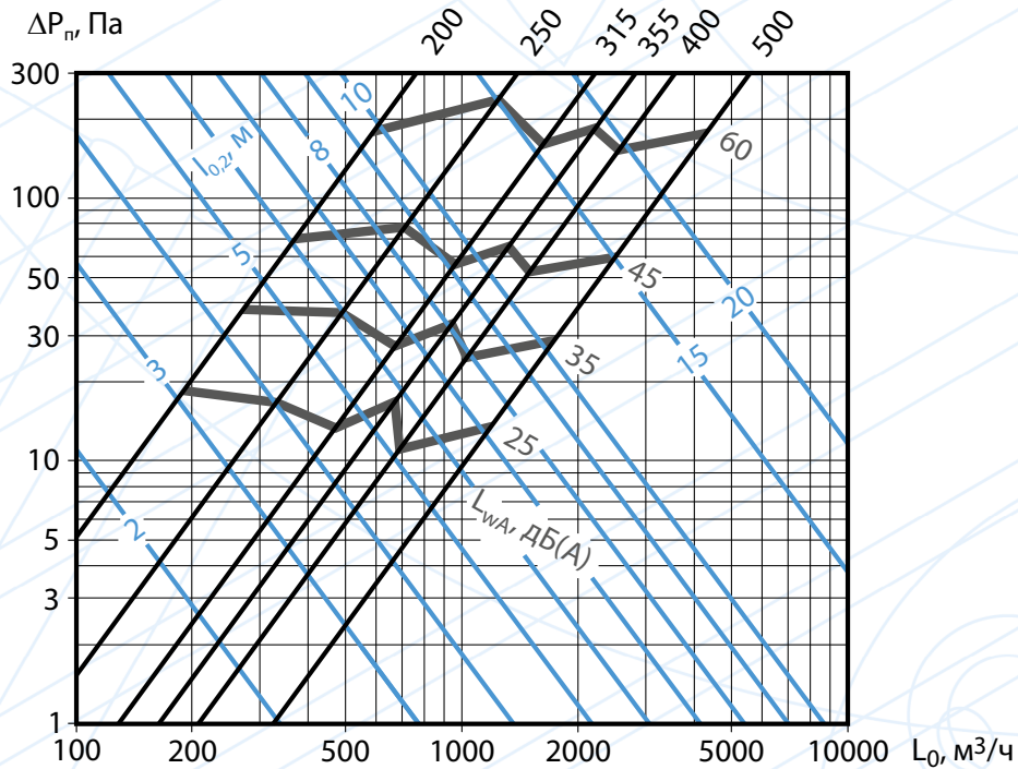
Аэродинамические и акустические характеристики ДКВ, ДКВ-Т при подаче воздуха в помещение веерной струей в свободных условиях при угле наклона лопаток \alpha=50^\circ
