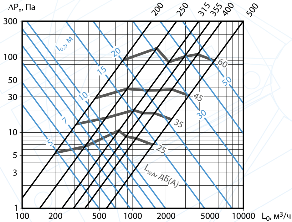
Аэродинамические и акустические характеристики ДКВ при подаче воздуха в помещение конической смыкающейся струей при угле наклона лопаток \alpha=30^\circ
