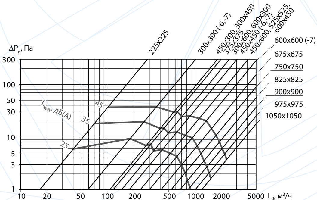
Аэродинамические и акустические характеристики диффузоров 4АПН, 4АПР при удалении воздуха из помещения
