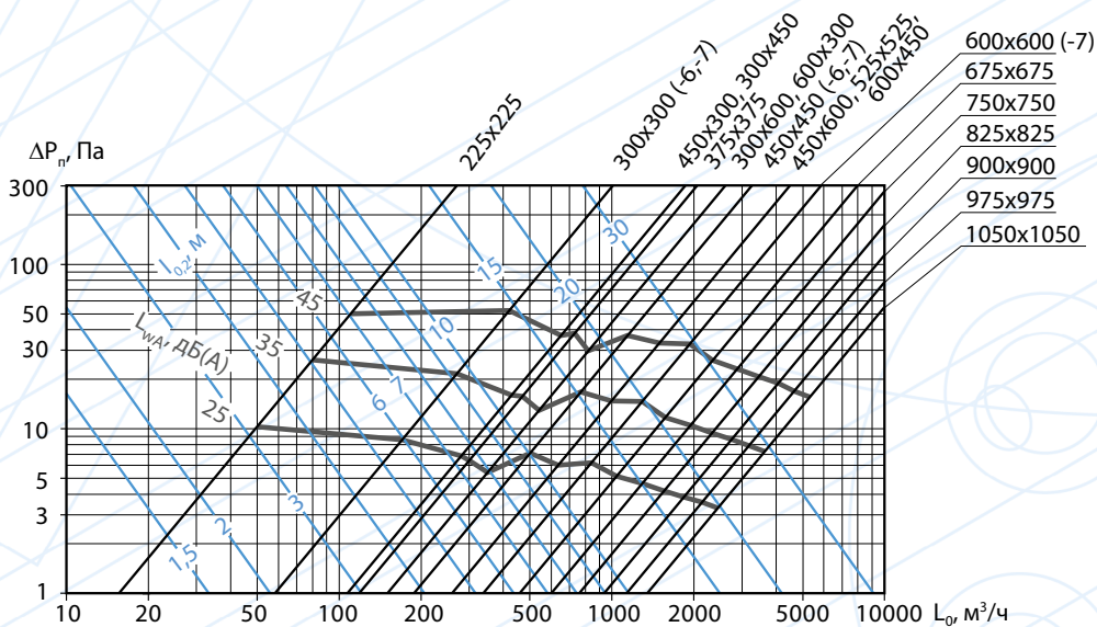
Аэродинамические и акустические характеристики диффузоров 4АПН, 4АПР при подаче воздуха в помещение четырехсторонними настиляющимися струями
