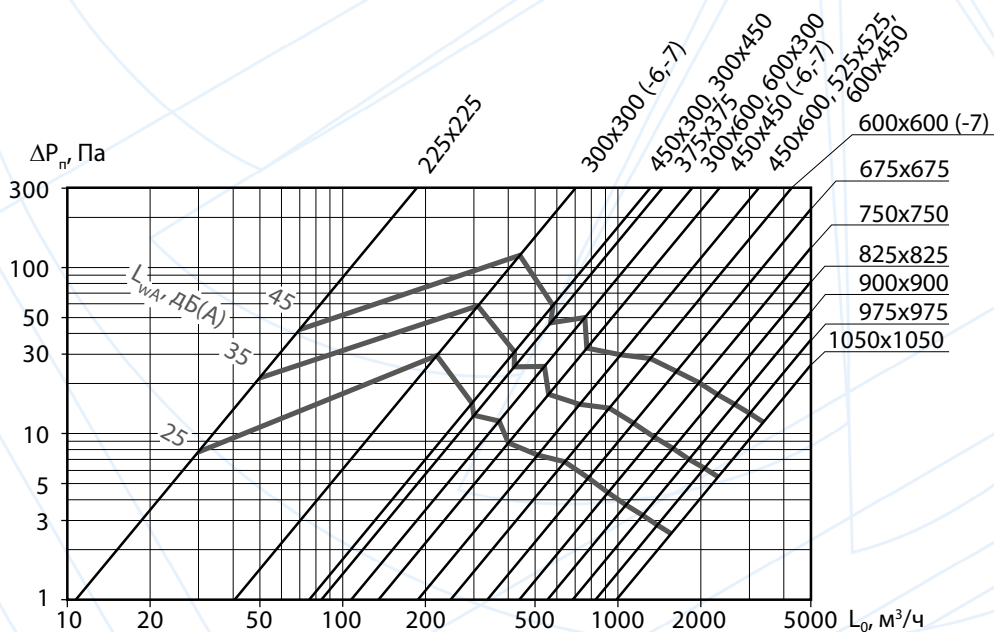
Аэродинамические и акустические характеристики диффузоров 1АПН, 1АПР при удалении воздуха из помещения
