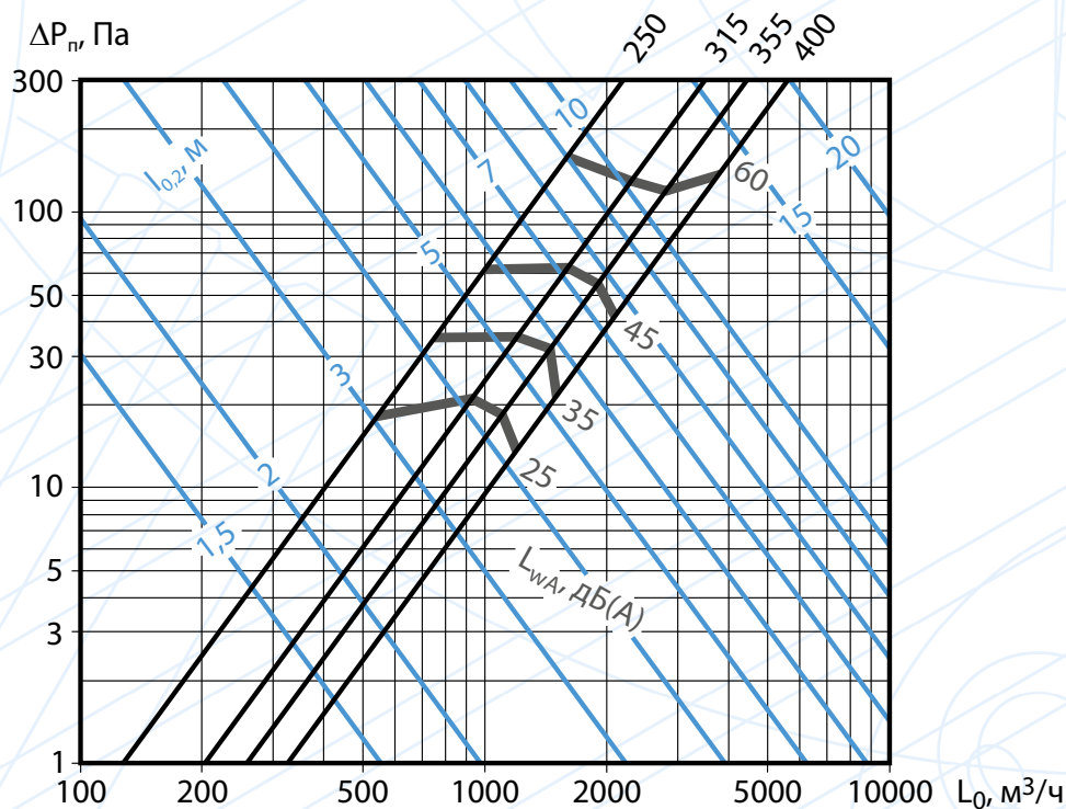
Аэродинамические и акустические характеристики диффузоров ДКУ (b=0 мм), 2ДКФ при подаче воздуха в помещение веерными струями в свободных условиях
