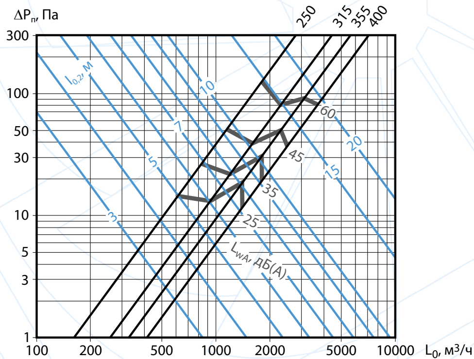
Аэродинамические и акустические характеристики диффузоров ДКУ, ДКК ( b > 0 мм) при подаче воздуха в помещение веерными настилающимися струями
