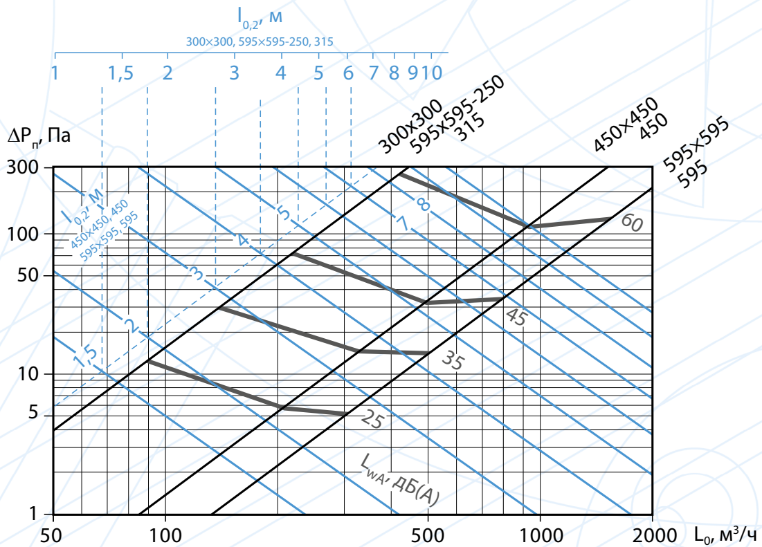
Аэродинамические и акустические характеристики 2ДПЗ М, 2ДКЗ М при подаче воздуха настилающейся верхней струей
