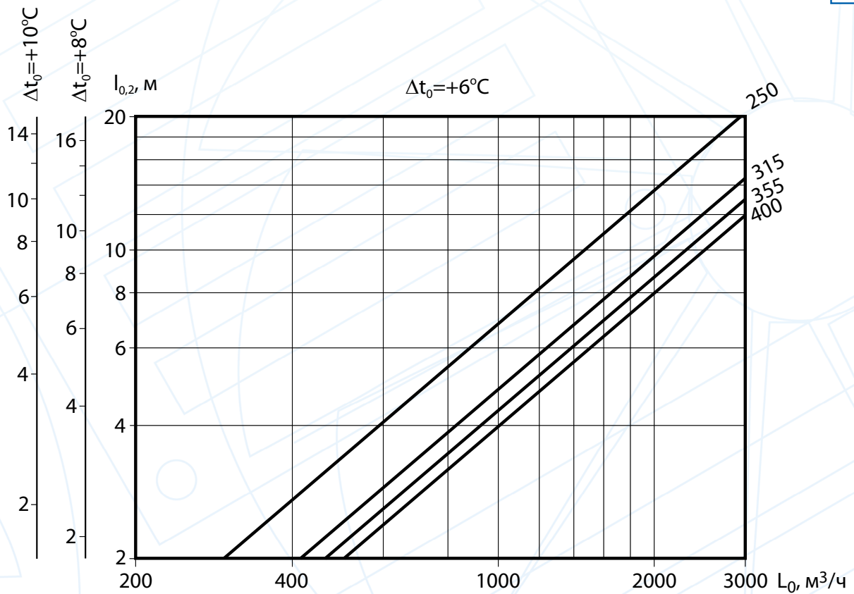
Дальность диффузоров ДКУ-Т, ДКК-Т при подаче воздуха в помещение неизотермическими вертикальными коническими струями при наличии поверхности настиления
