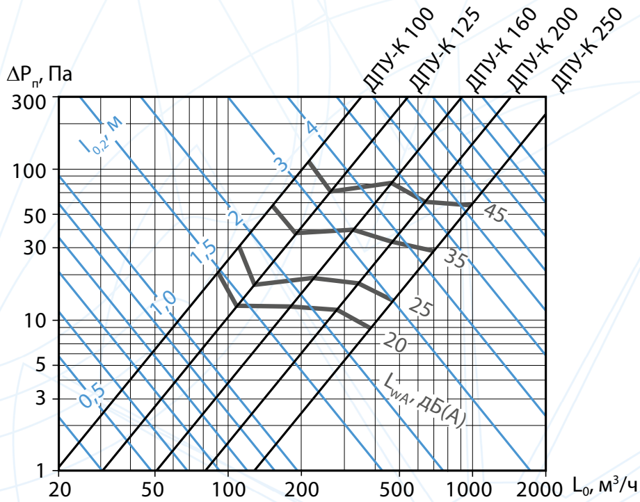
Аэродинамические и акустические характеристики ДПУ-К (b=0,05A) при подаче воздуха в помещение настилающимися верными струями
