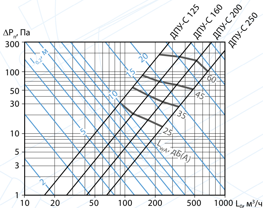
Аэродинамические и акустические характеристики ДПУ-С при подаче воздуха в помещение
