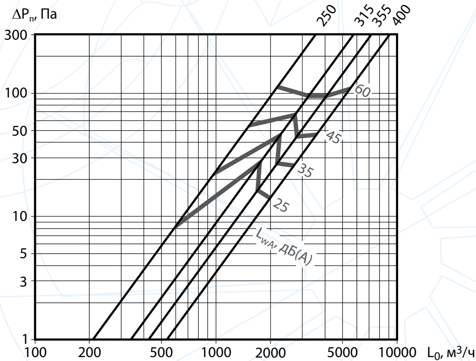
Аэродинамические и акустические характеристики диффузоров ДКУ, ДКК (b=0 мм), 2ДКФ при удалении воздуха из помещения
