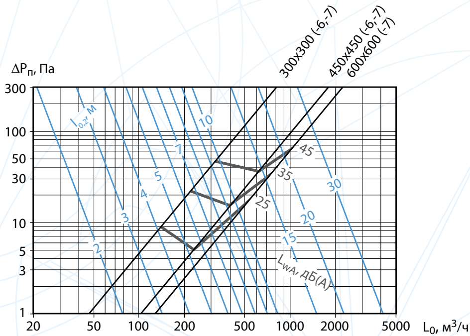
Аэродинамические и акустические характеристики диффузоров 1АГН, 1АГР при подаче воздуха в помещение четырехсторонним настилающимся потоком
