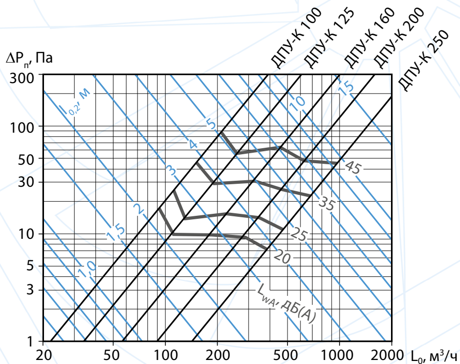
Аэродинамические и акустические характеристики ДПУ-К (b=0,1A) при подаче воздуха в помещение коническими струями
