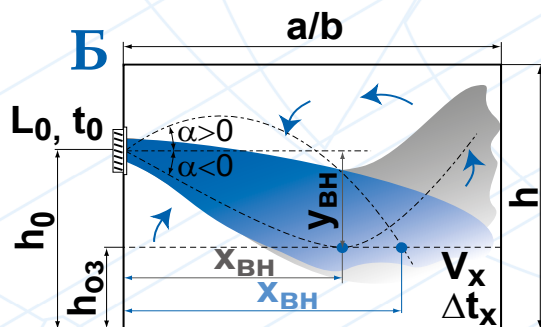
Схема Б Подача воздуха сверху вниз наклонными струями
