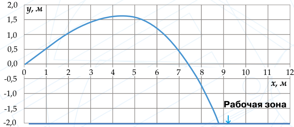
Рисунок Б1 - Траектория развития холодной струи
