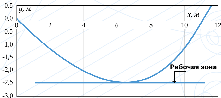
Рисунок Б2 - Траектория развития теплой струи
