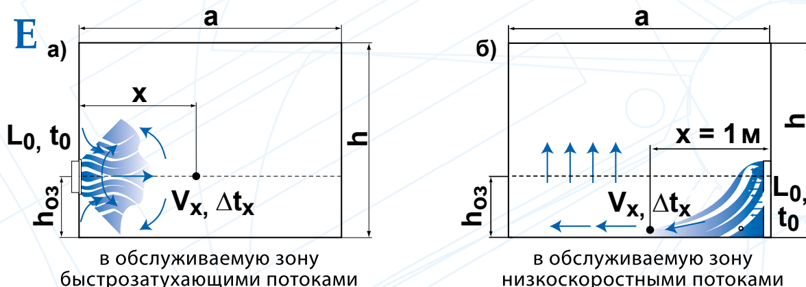
Схема Е Подача воздуха в рабочую зону быстрозатухающими и низкоскоростными потоками
