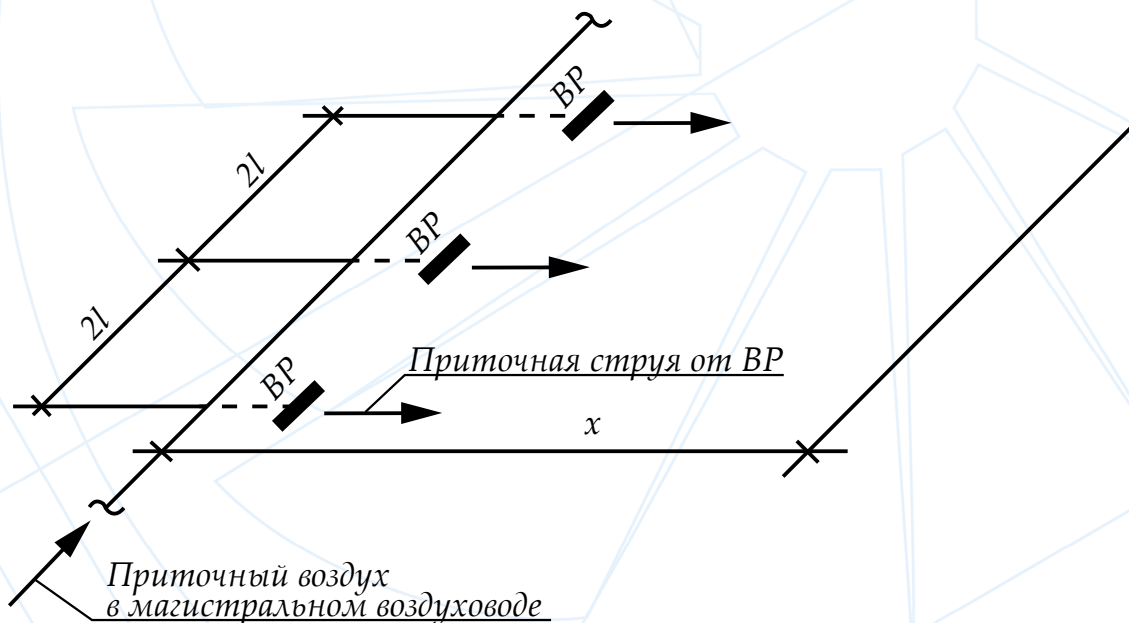
Рисунок П.1 - Схема установки ВР в ряд
