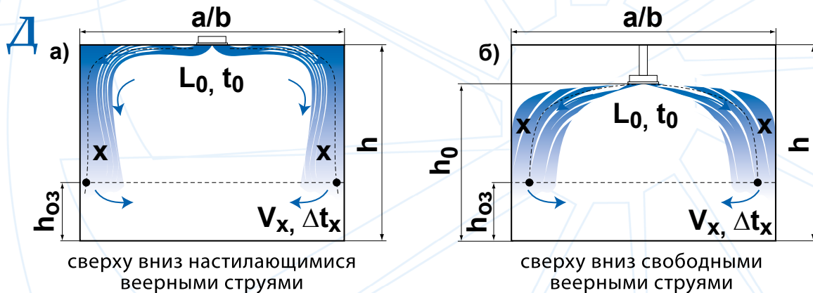
Схема Д Подача воздуха сверху вниз веерными струями
